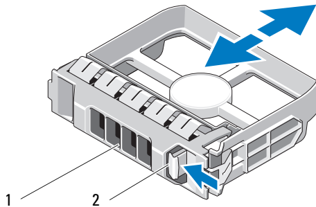
图 16-2. 卸下和安装 3.5 英寸硬盘驱动器挡片（仅限 MD3600f）
